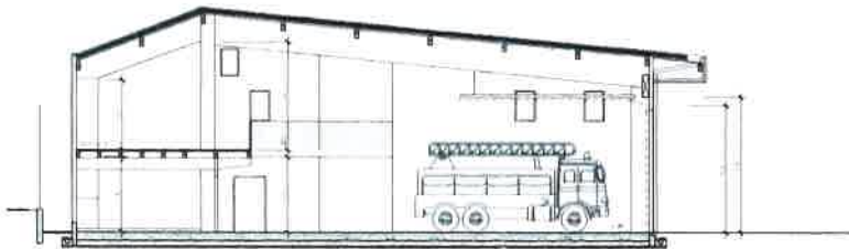
COUPE HALLE VEHICULE
