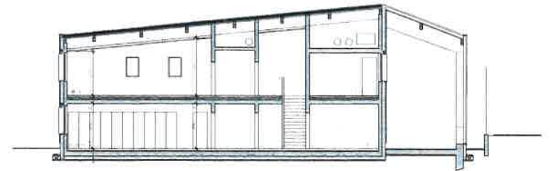
COUPE ENTREE
